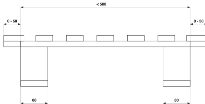
b.) ≤ 500 mm 2 Palettenfüße alle Angaben in mm Einfahrseite - großes Maß
