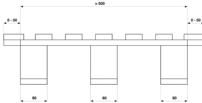
a.) > 500 mm 3 Palettenfüße alle Angaben in mm Einfahrseite - großes Maß
